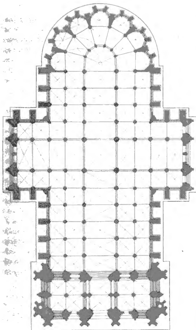
DOM VON KÖLN. GRUNDFISS.
